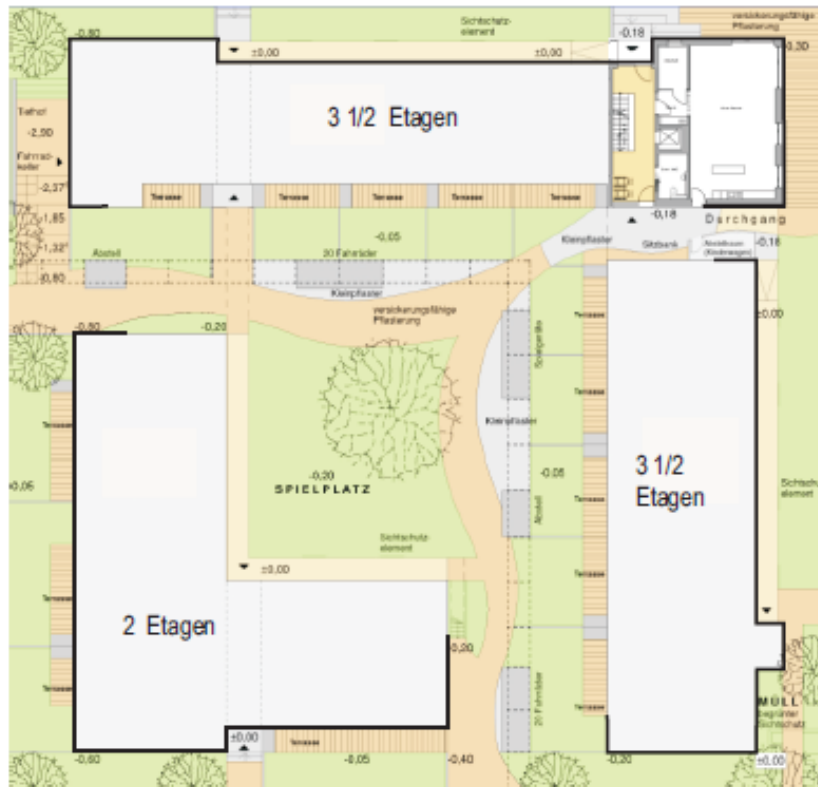
Freiflächenplan
