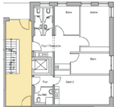
Home Office und Gästeapartment 2 im 2. Obergeschoss
